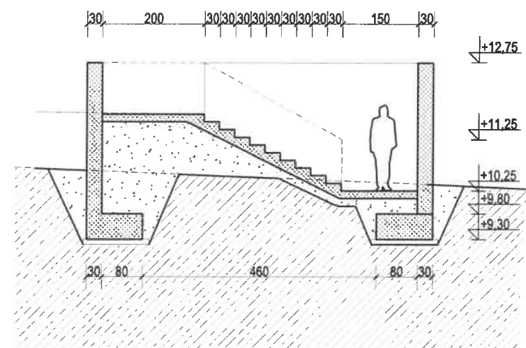
PRESJEK 2-2
