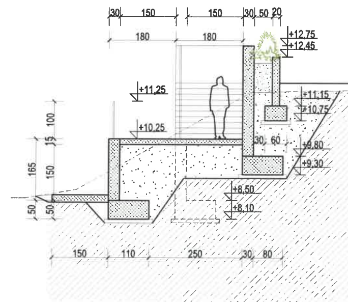
PRESJEK 3-3
