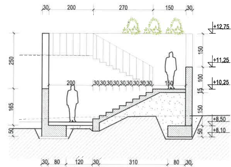
PRESJEK 1-1
