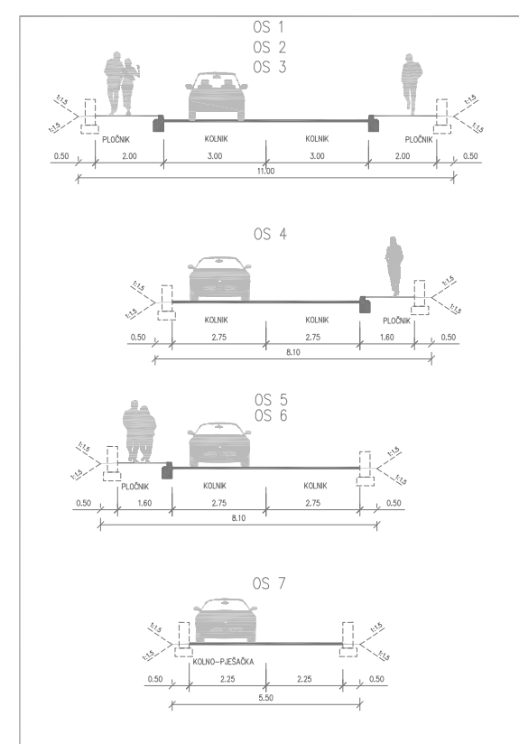
Karakteristični normalni presjeci kolnih prometnica M 1:200
