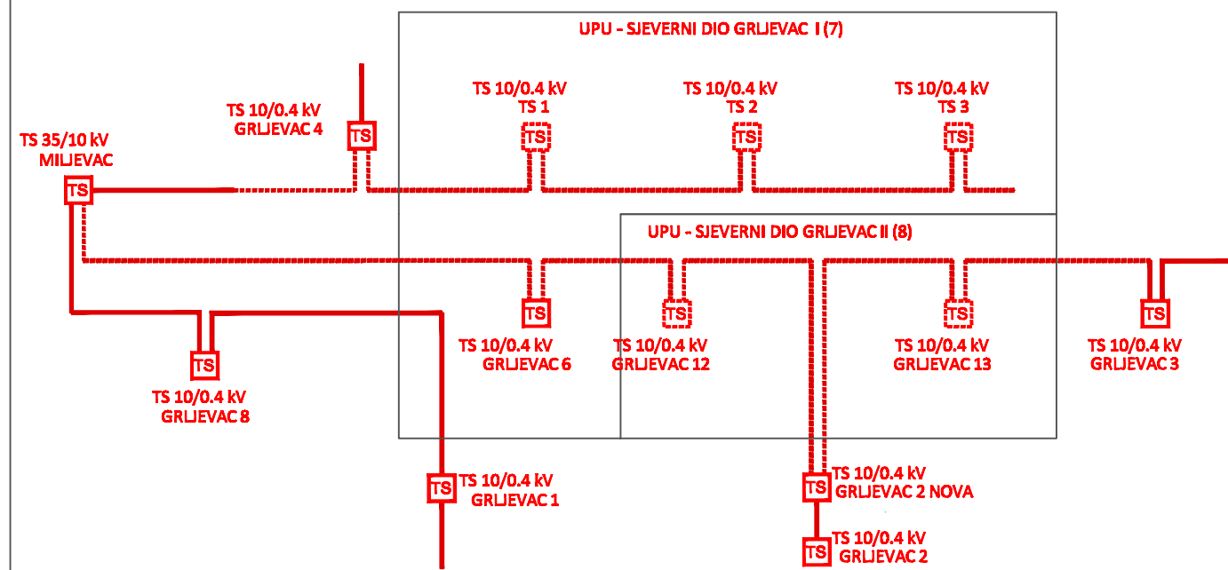
HEMA UKLAPANJA PLANIRANIH TS 10/0.4 KV U POSTOJEĆU 10 KV MREŽU
